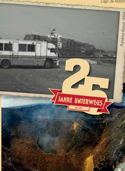
Vulkan Masaya, Nicaragua
